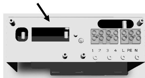
Stecken Sie den RJ45-Stecker in den dafür vorgesehenen RJ45-Steckplatz
