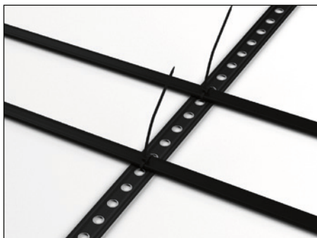
Montagelochband (Stahlblech, kunststoffumman- telt) als Abstandshalter bei Mehrfachverlegung. Typ: MLB-10
