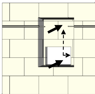
Leerrohr Größe M20 unterhalb des Fortluftrohres zur Kabeleinführung des Wandeinbaukastens
