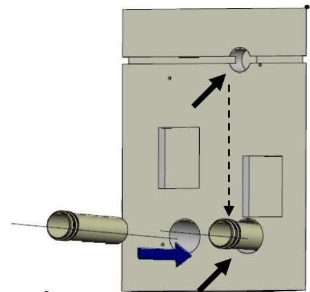
Kabelschlitz vom Kabelauslass (oben) zum Fortluftrohr für Leerrohr Größe M 20. Das Leerrohr ist unterhalb des Fortluftrohres nach außen zu führen.
