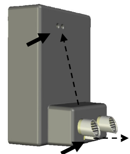
Leerrohrverlauf hinter Wandeinbaukasten
