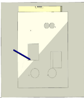
Zwei Kabelausslässe lt. Bohrschablone (für Zuleitung und Lüftungsgitterbeheizung)
