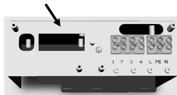
Stecken Sie den RJ45-Stecker in den dafür vorgesehenen RJ45-Steckplatz
