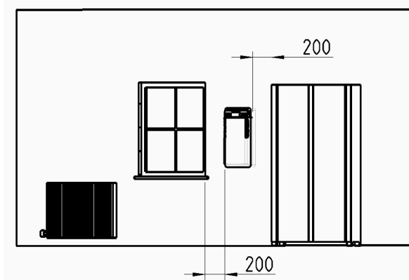
Montage mit Bedienfeld auf Augenhöhe Maßangaben sind Mindestabstände
