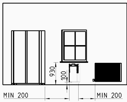
Montage unterhalb vom Fenster Maßangaben sind Mindestabstände
